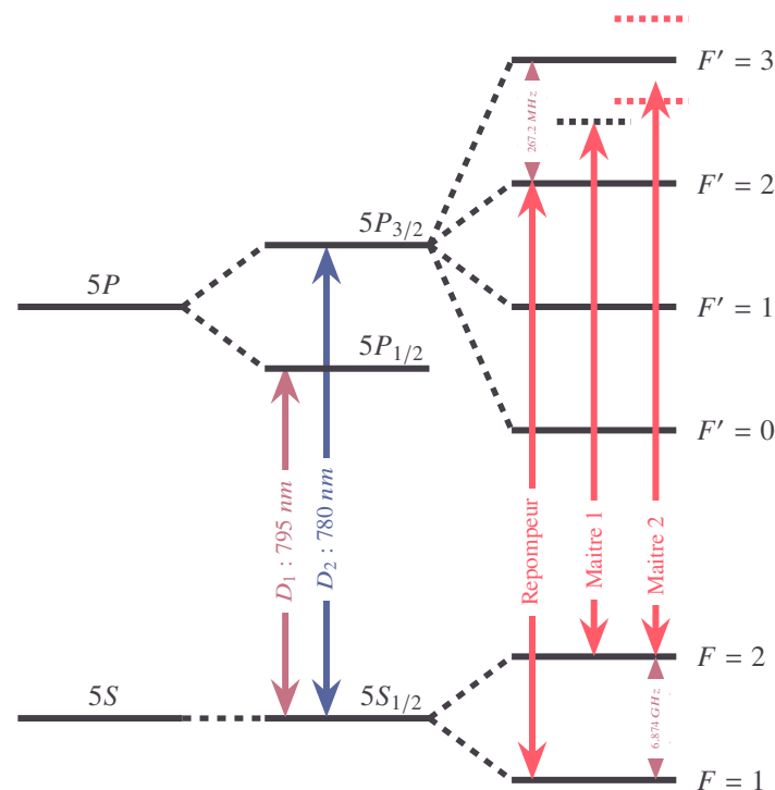
FIGURE V.1 – Structure hyperfine (transitions D1 et D2) de l'atome de Rubidium ^{87}\text{Rb} . Les longueurs d'onde des différents lasers utilisés dans l'expérience sont représentées en rouge vif
